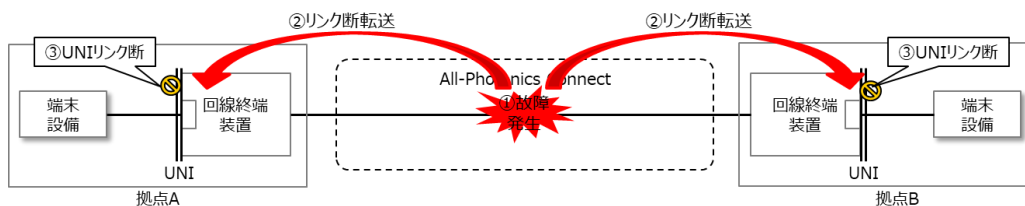
図 2-3-2 リンク断転送機能(網内)の動作 ※
