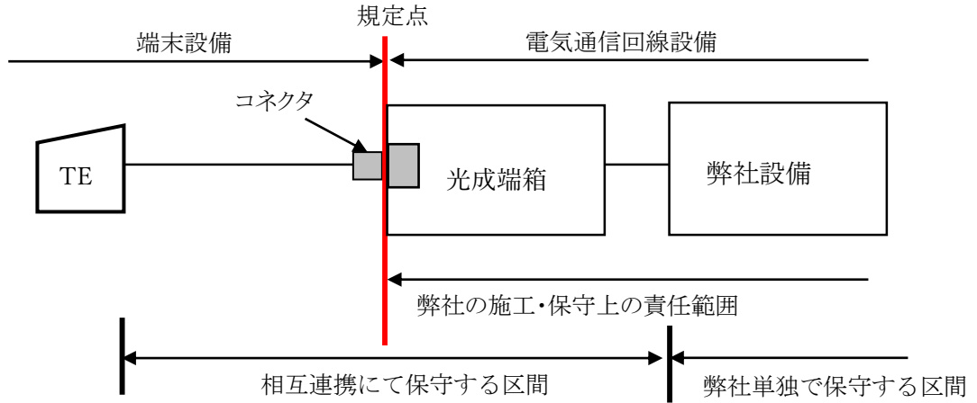
図 3-1-3 All-Photonics Connect の UNI 規定点(光成端箱)
