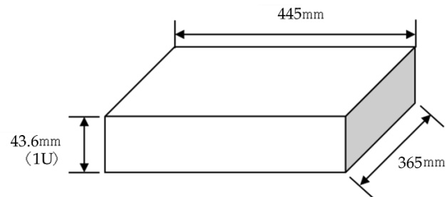
図 4-1-3 コンバータ
