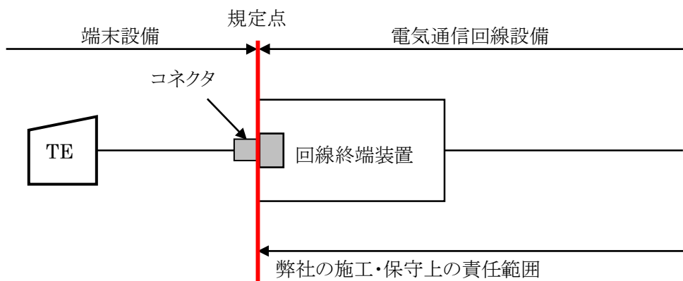
図 3-1-1 All-Photonic Connect の UNI 規定点 (装置終端)
