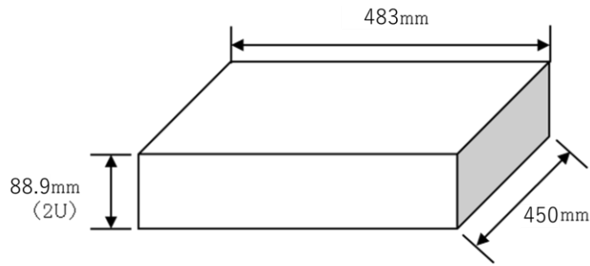
図 4-1-2 回線終端装置外観(DC 電源)
