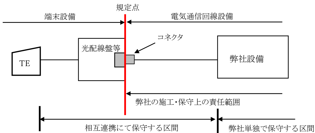
図 3-1-2 All-Photonic Connect の UNI 規定点 (コネクタ終端)
