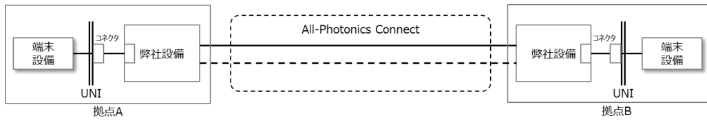
図 2-4-1 中継区間冗長化メニュー
