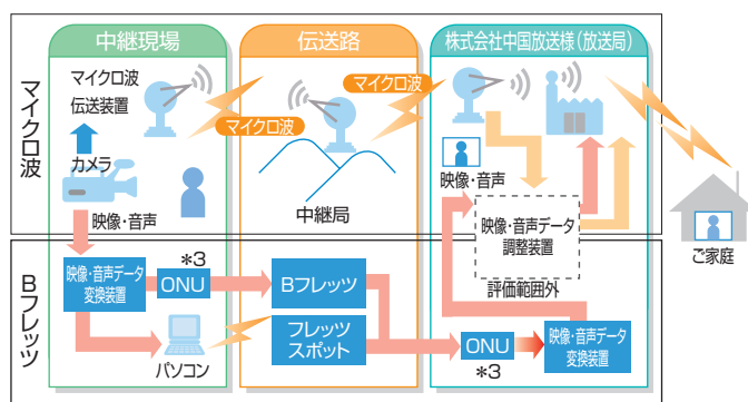
Bフレッツを用いたTV中継システム(マイクロ波を用いたシステムとの比較)
